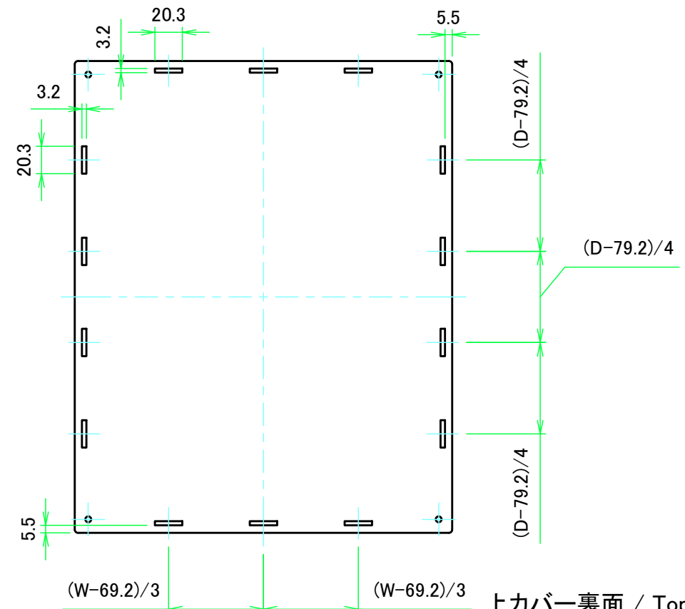
上カバー裏面 / Top cover Backside
